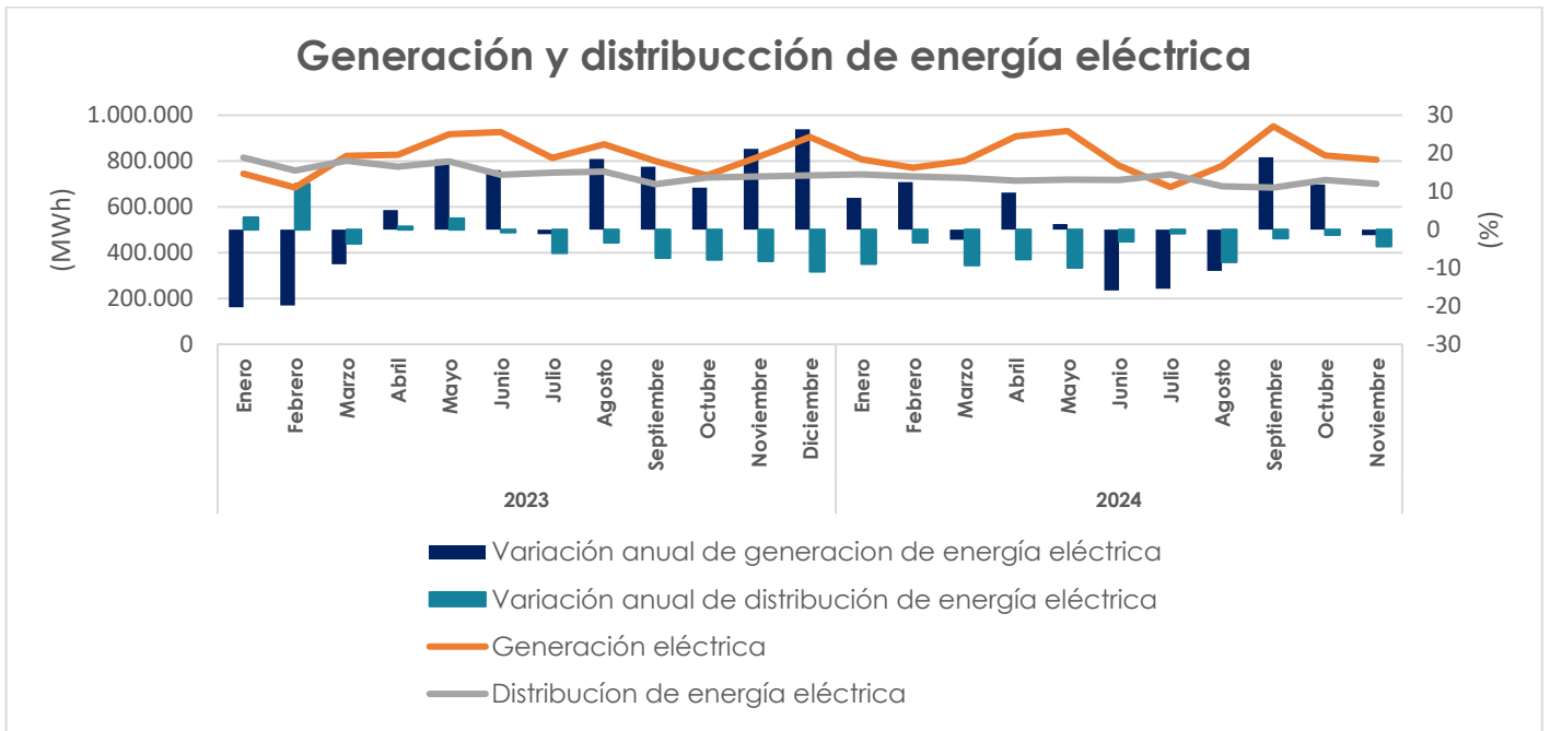
Gráfico 18. Generación eléctrica y distribución de energía eléctrica región de Atacama. INE
